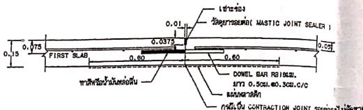
รูปขยายรอยต่อ CONSTRUCTION JOINT และ CONTRACTION JOINT
