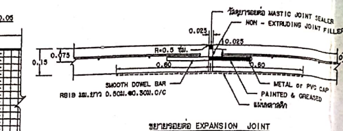
รูปขยายรอยต่อ EXPANSION JOINT
