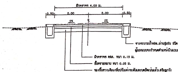
รูปตัดถนนคอนกรีตเสริมเหล็ก (กรณีจราจรระบายน้ำ)
